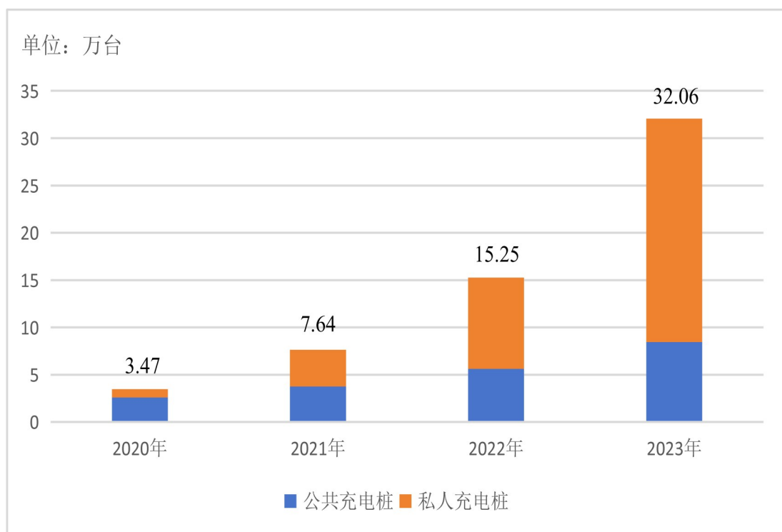
图2 2020—2023 年四川省充电基础设施保有量情况
